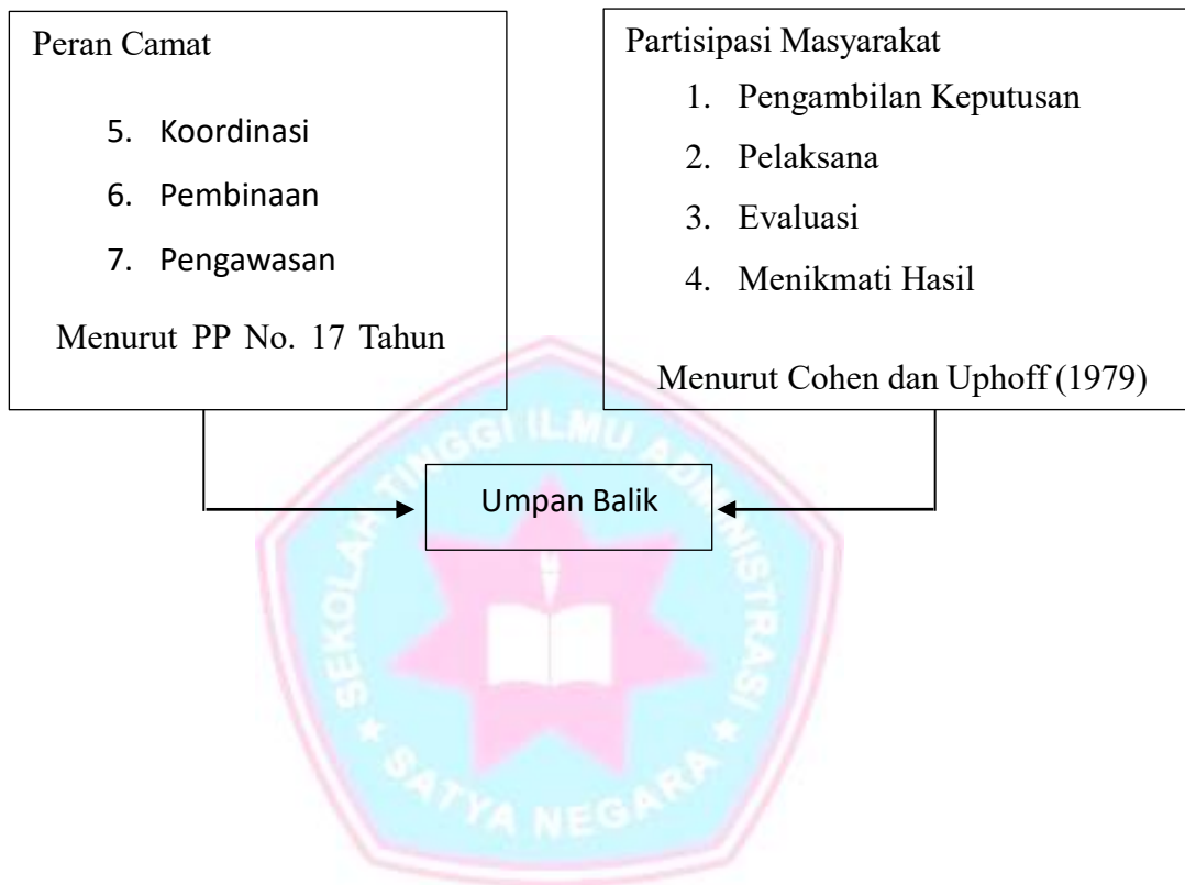
Gambar 1 Kerangka Berpikir
